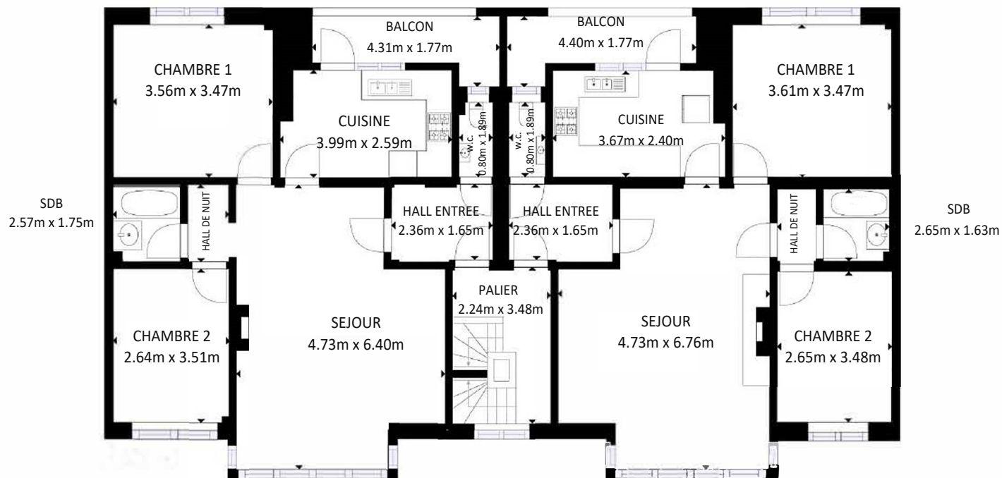
1er ETAGE
